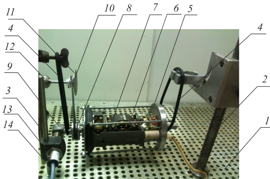
Рис. 1. Экспериментальная установка
